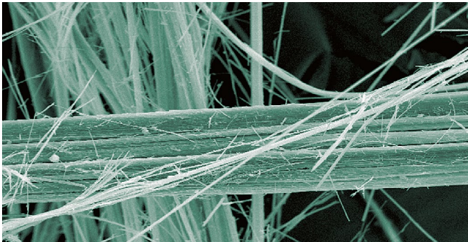
Asbestfasern 1/10 mm
